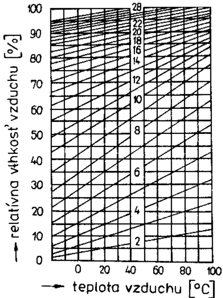
Graf rovnovážnej vlhkosti dreva
